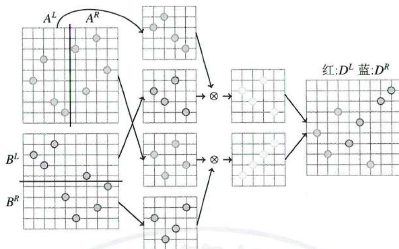
图 1: 分治得到 D^L, D^R 的过程
